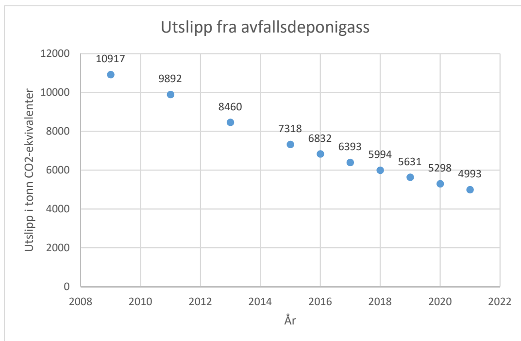
Figur 16 - Utslipp fra avfallsdeponigass
