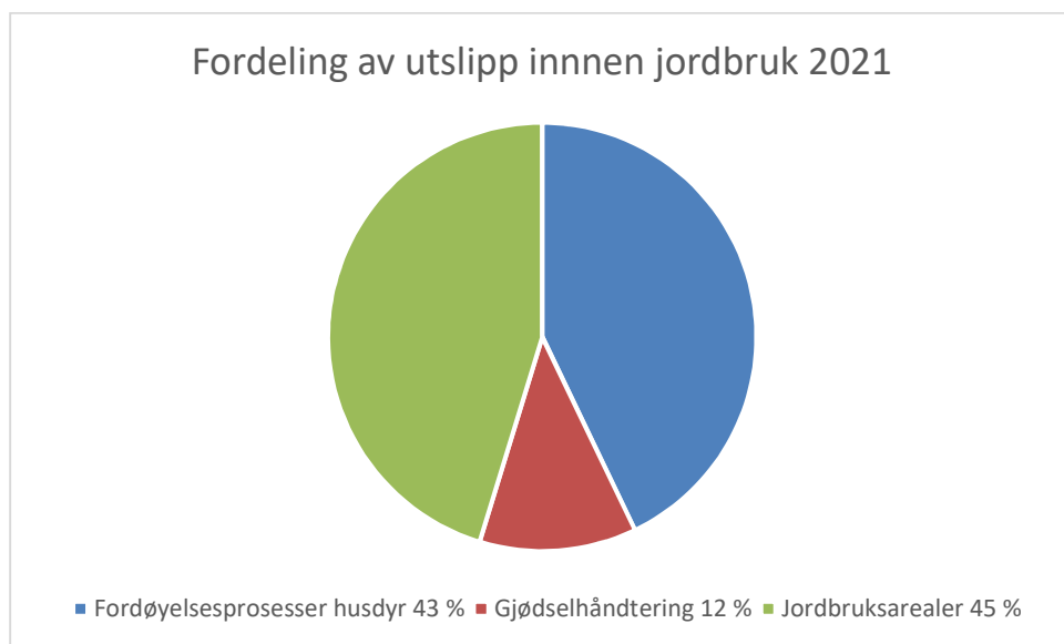
Figur 13 - Fordeling av utslipp fra sektoren jordbruk i 2021
