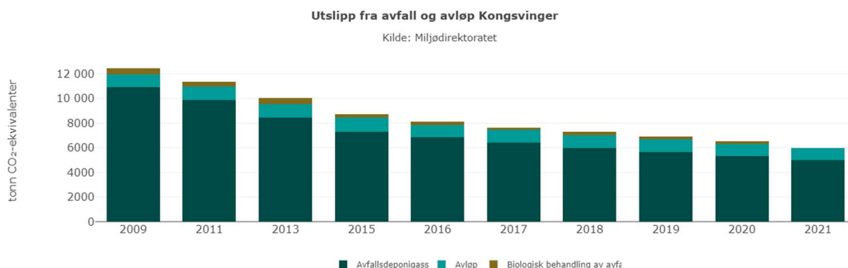
Figur 14 - Utslipp fra sektoren avfall og avløp i perioden 2009 – 2021
