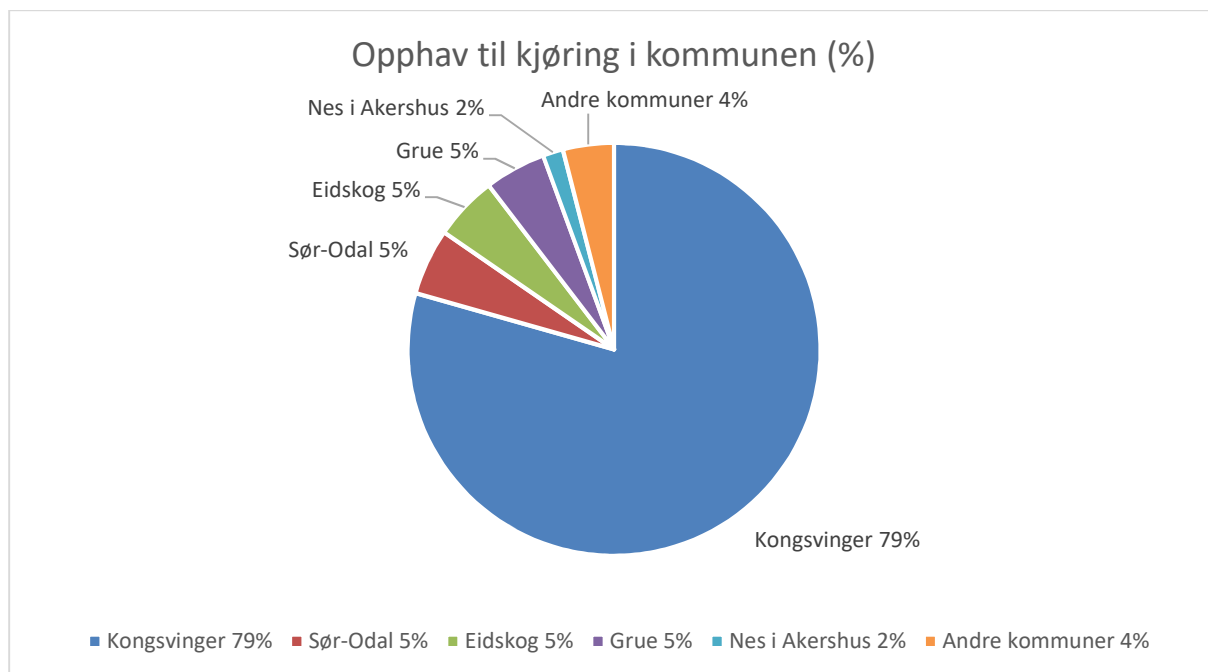
Figur 7 - Fordelingen av opphavet til kjøring i Kongsvinger kommune i 2016
