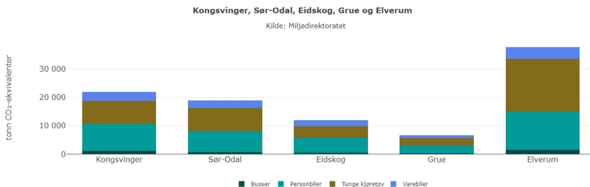
Figur 24 - Utslipp fra veitrafikk i 2021
