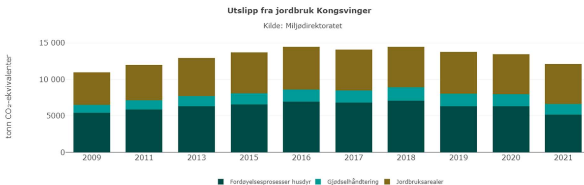
Figur 12 - Utslipp fra sektoren jordbruk i årene 2009 – 2021
