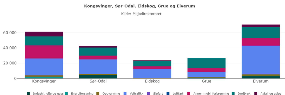
Figur 23 - Utslipp totalt per kommune i tonn CO 2 -ekvivalenter i 2021
