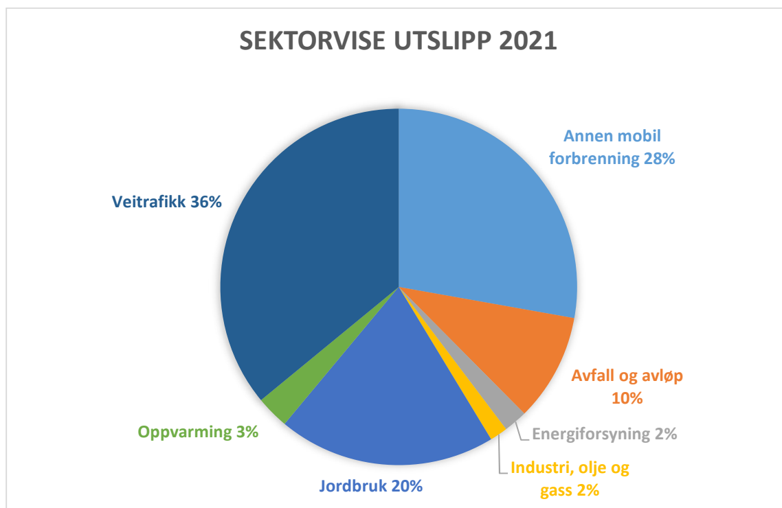
Figur 2 - Fordeling av utslippene i 2021
