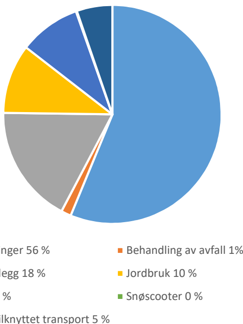
Figur 9 - Fordeling av utslippene fra annen mobil forbrenning i 2021
