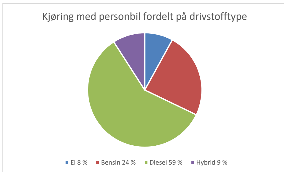
Figur 5 - Kjøring med personbil fordelt på drivstofftype i 2021 i Kongsvinger kommune
