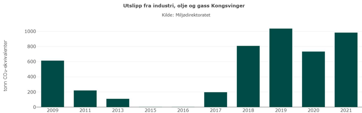
Figur 22 - Utslipp fra sektoren industri, olje og gass i Kongsvinger i perioden 2009 - 2021
