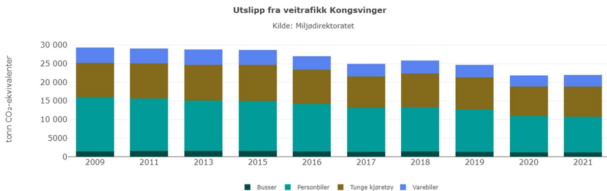
Figur 3 - Utslipp fra veitrafikk i årene 2009 – 2020
