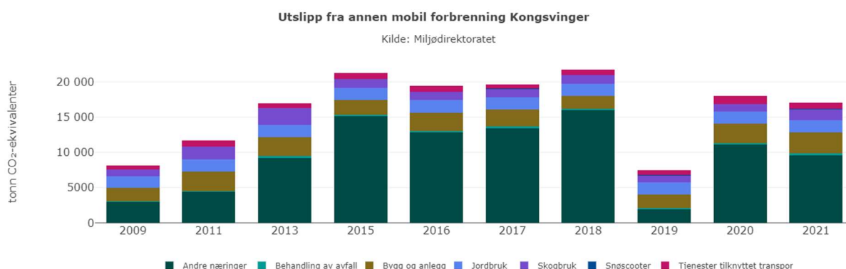
Figur 8 - Utslipp fra sektoren annen mobil forbrenning i årene 2009 – 2021.
