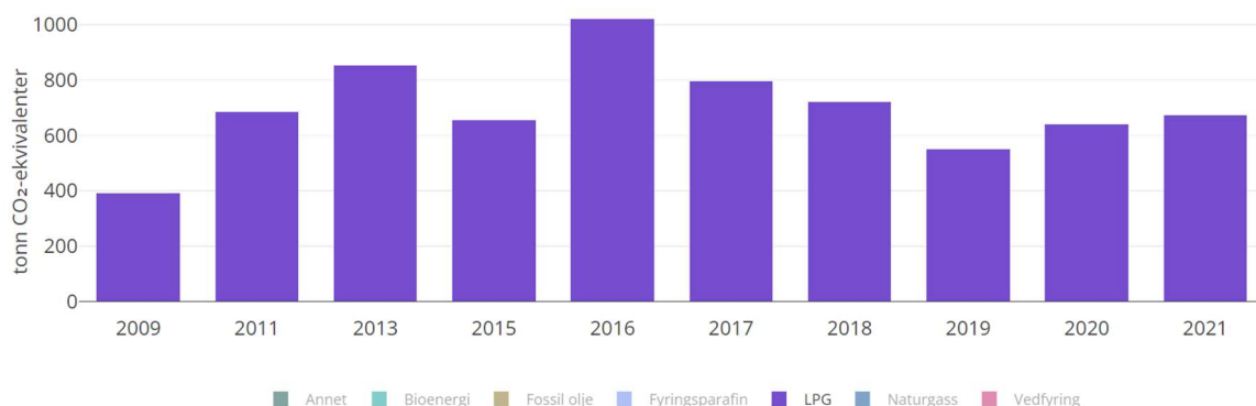
Figur 18 - Utslipp fra LPG i Kongsvinger kommune i perioden 2009 – 2021
