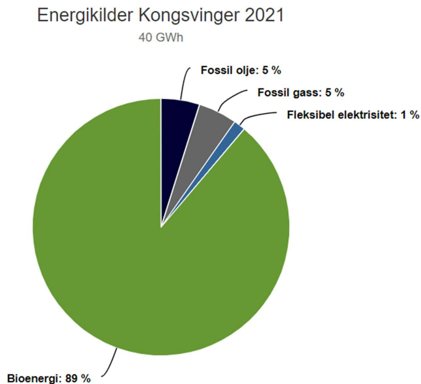
Figur 20 - Energikilder for fjernvarme i Kongsvinger 2021
