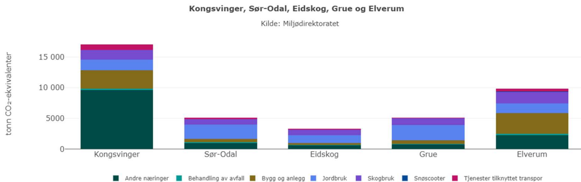
Figur 25 - Utslipp fra annen mobil forbrenning i 2021
