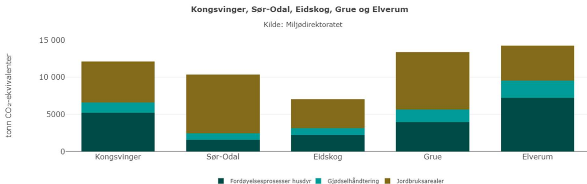
Figur 26 - Utslipp fra jordbruk i 2021
