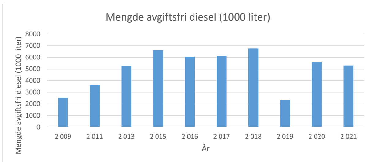
Figur 11 - Mengde avgiftsfri diesel (1000 liter).
