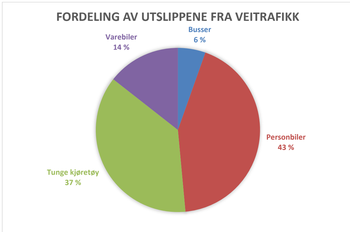
Figur 4 - Fordeling av utslippene fra sektoren veitrafikk
