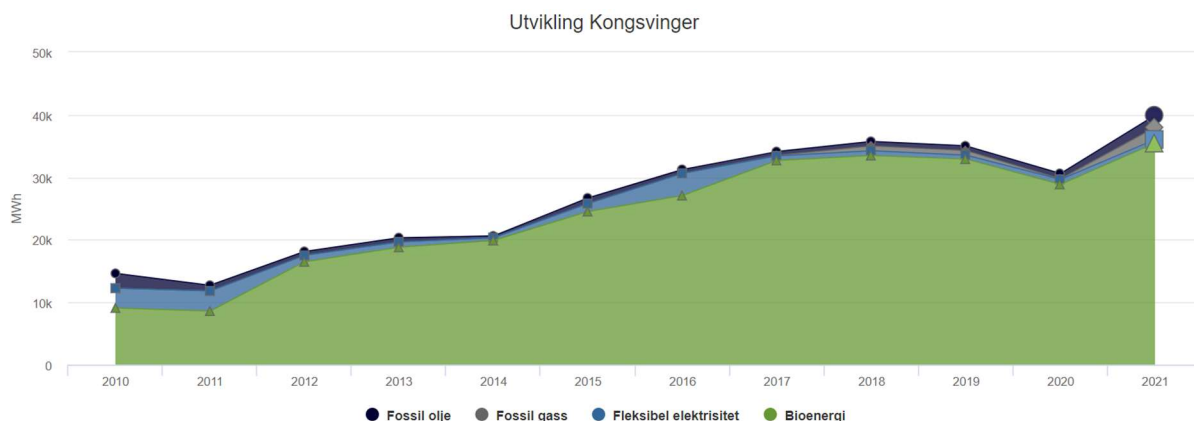
Figur 21 – Utvikling av energikilder over tid i Kongsvinger
