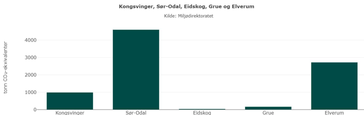
Figur 30 - Utslipp fra industri, olje og gass i 2021
